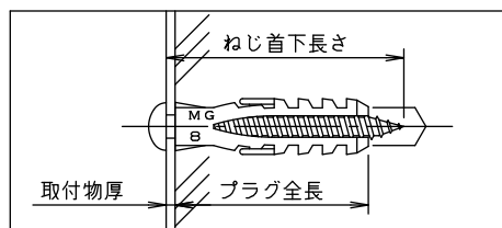
取付寸法図
