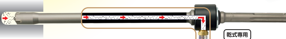
集塵機
