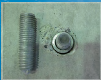
引張試験後の破壊状況
