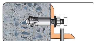
④取付け(所定のトルク値で施工してください)
