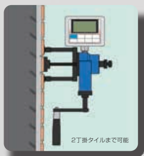
外壁タイルの引張荷重確認
