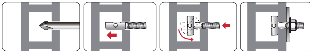
① 穿孔 取付け
